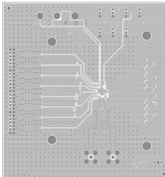
Inner Layer 3
